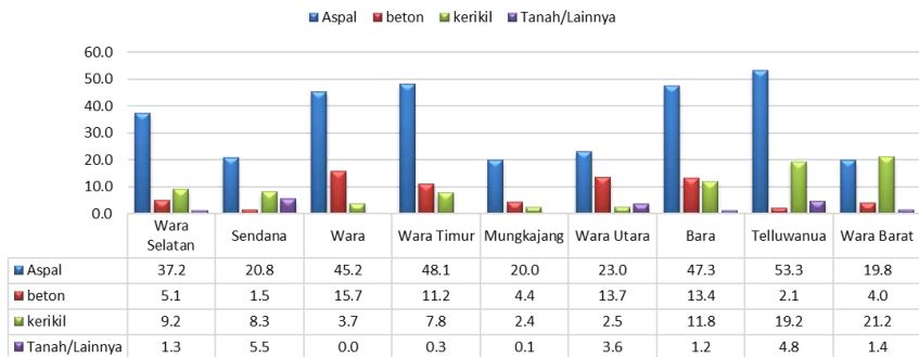
Gambar 5. 8 Panjang Jalan (km) Menurut Jenis Permukaan Jalan dan Kecamatan di Kota Palopo Tahun 2024
